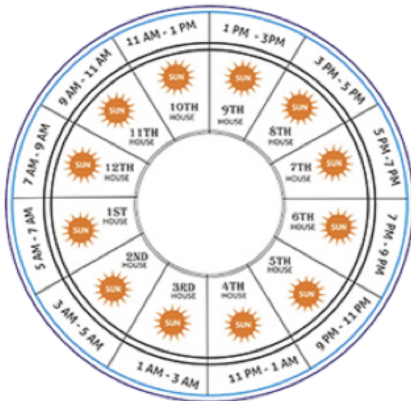
Il Sole transita attraverso le 12 case e le diverse ore del giorno
